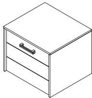
5202-WAG-U-001 szafka umywalkowa 600x490x535
