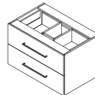
5103-WAG kontener pod umywalkę 800x500x525
