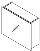
5208-WAG szafka wisząca - lustro 600x468x182
